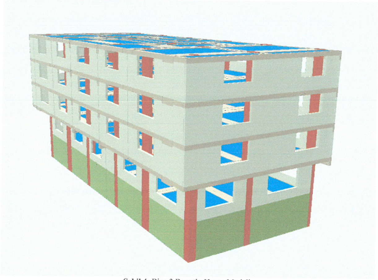
Şekil 4: Bina 3 Boyutlu Hesap Modeli
